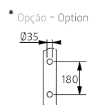
Pormenor da ába - Rim detail
